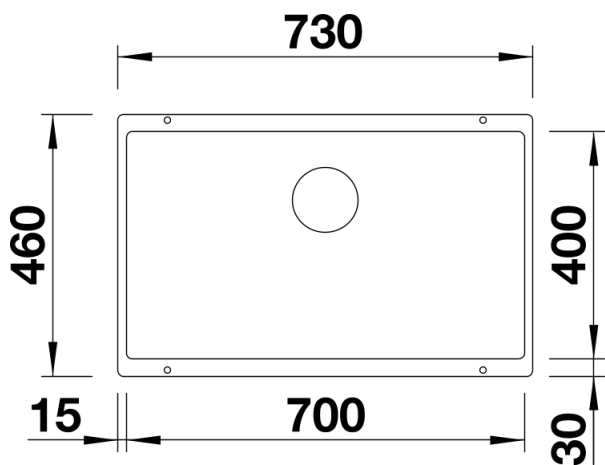
Aufsicht
