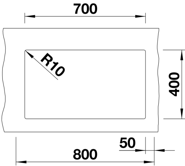
Ausschnitt
